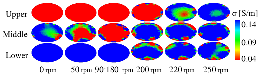
図8 各回転数ならびに各断面におけるトモグラフィー画像
